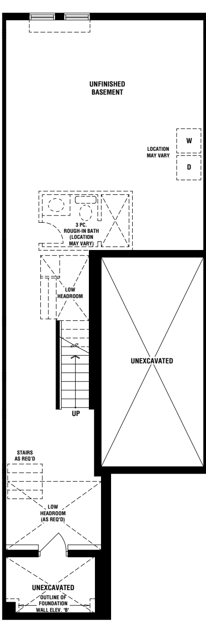
BASEMENT ELEV. 'A' & 'B'
